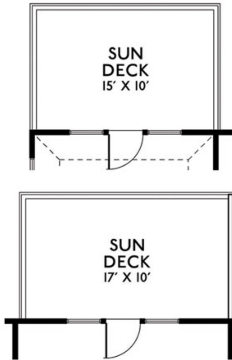
Optional Back Porches
